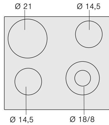
PKN6..F17.
