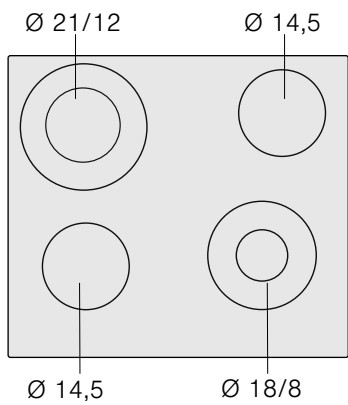
PKG6..F17., PKG6..FB1.
