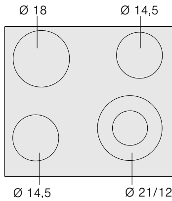
PKF65.F17., PKF67.F17.
