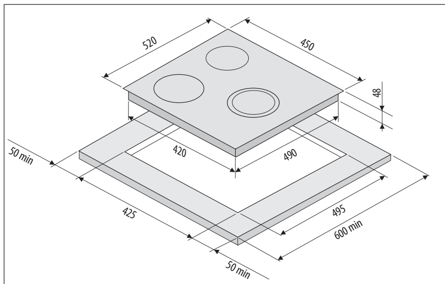
Схема встраивания варочной поверхности FIDATO 45 BL
