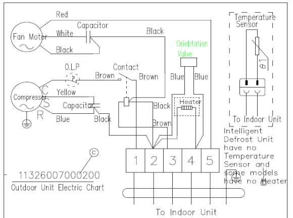
Наружный блок моделей RAS/RAC-24N2X
