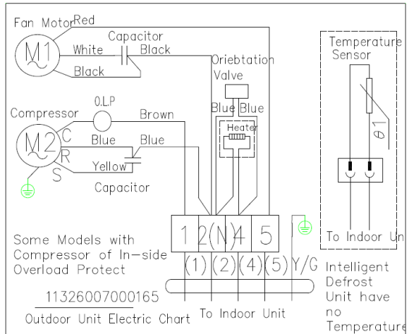
Наружный блок моделей RAS/RAC-24N2X
