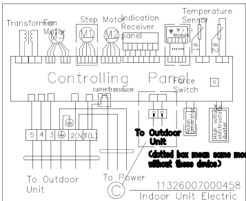
Внутренний блок модели RAS/RAC-24N2X
