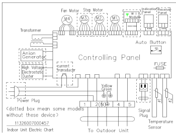
Внутренний блок модели RAS/RAC-24N2X
