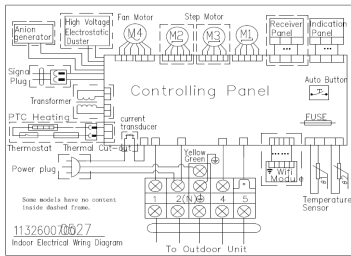
Внутренний блок моделей RAS/RAC-12N2X, 18N2X
