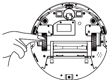
Очистка правого и левого колеса
