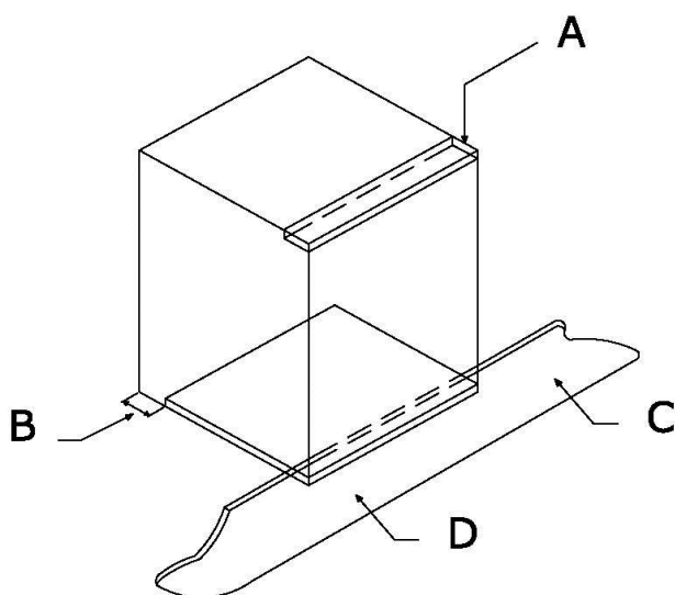
Рис. 7. Указания по вентиляции и зазорам при установке простой электродуховке в стандартный кухонный блок.
