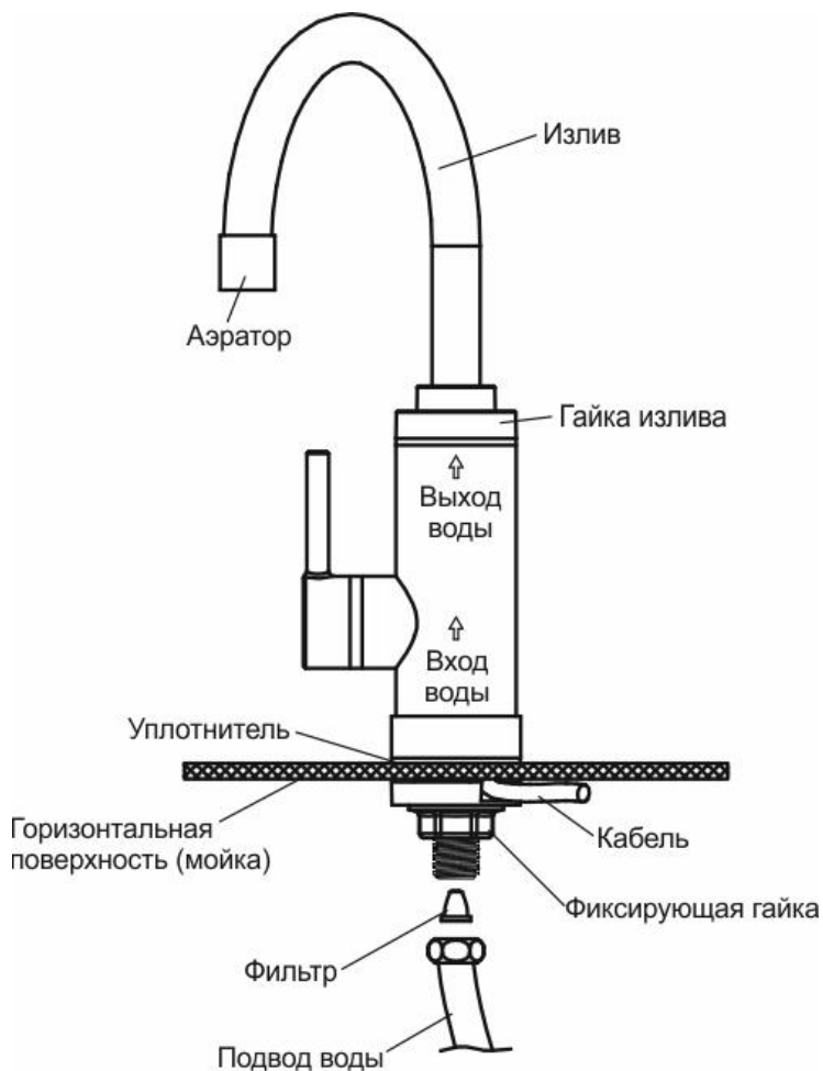
Рис. 1. Схема ПЭВН Thermex Hotty 3000
