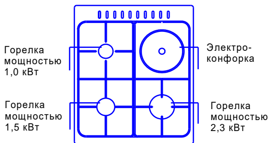
Рис. 16. Верхняя панель плит ЭГ1/3г01МС-2у; ЭГ1/3г01М2С-2у; ЭГ1/3г14МС-у; ЭГ1/3г14М2С-2у;
