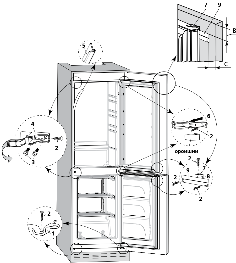
Расми 8 – Нақшаи мустанкам кардани яхдони дохили мебел
