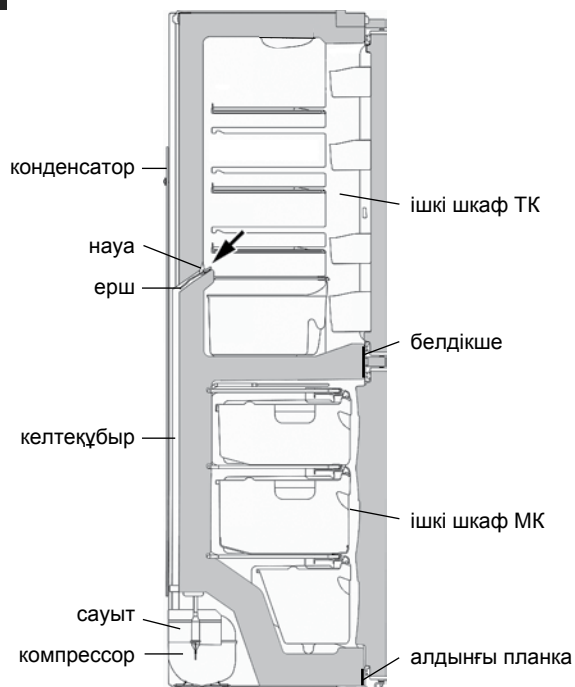
10 сурет – Еріген суды ағызу схемасы
