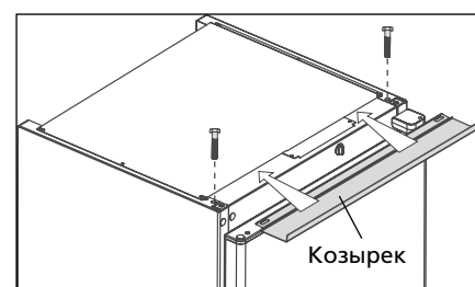
Сурот 7 – Козырөктү орнотуу
