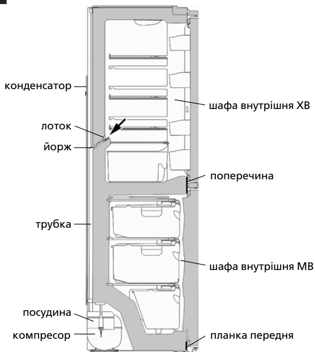
Рисунок 10 – Схема зливу талої води
